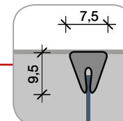
pvc profiel 1 demonteerbaar
