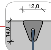
pvc profiel 2 demonteerbaar
