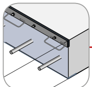
Splitboard® met dwarskracht overdracht
