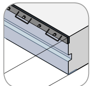
bijkomende vertanding
