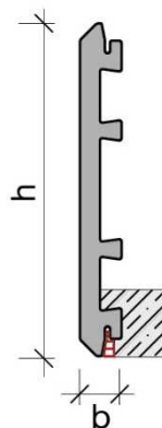
Wersja do płyt z listwą uszczelniającą (AKZ-D)
