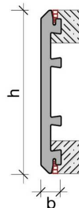
Wersja do ścian z dwoma listwami uszczelniającymi (AKZ-W)
