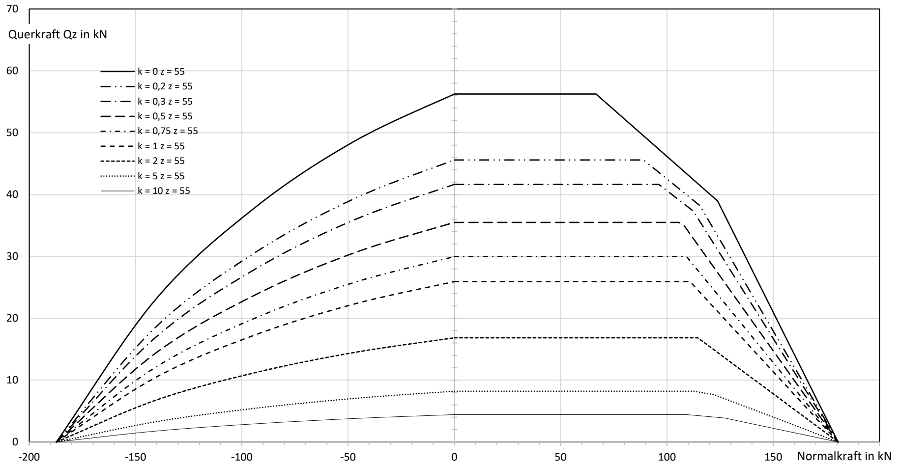
Abb. 6: Querkraft in z-Richtung, FVST 16, z = 55 mm
