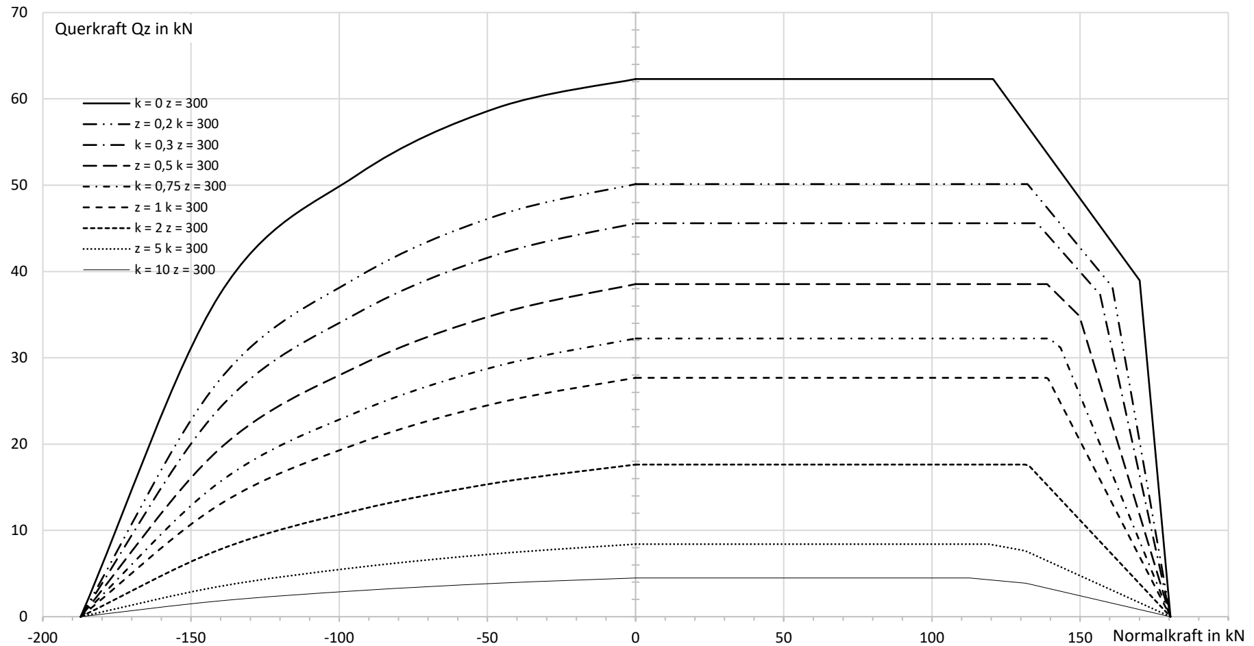
Abb. 8: Querkrft in z-Richtung, FVST 16, z = 300 mm
