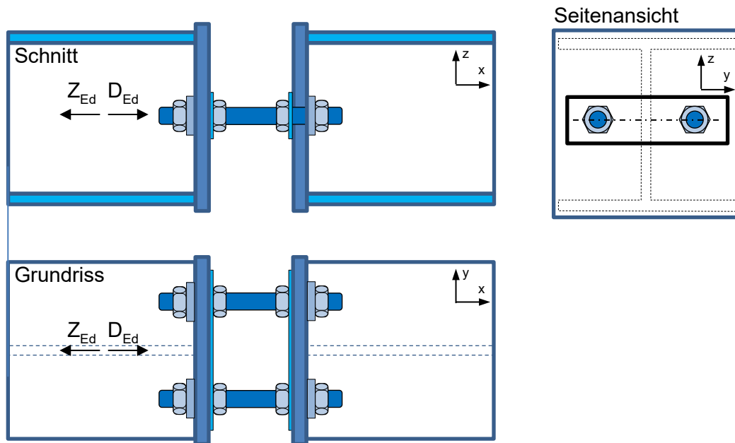
Abb. 1: Ein Modul FZST
