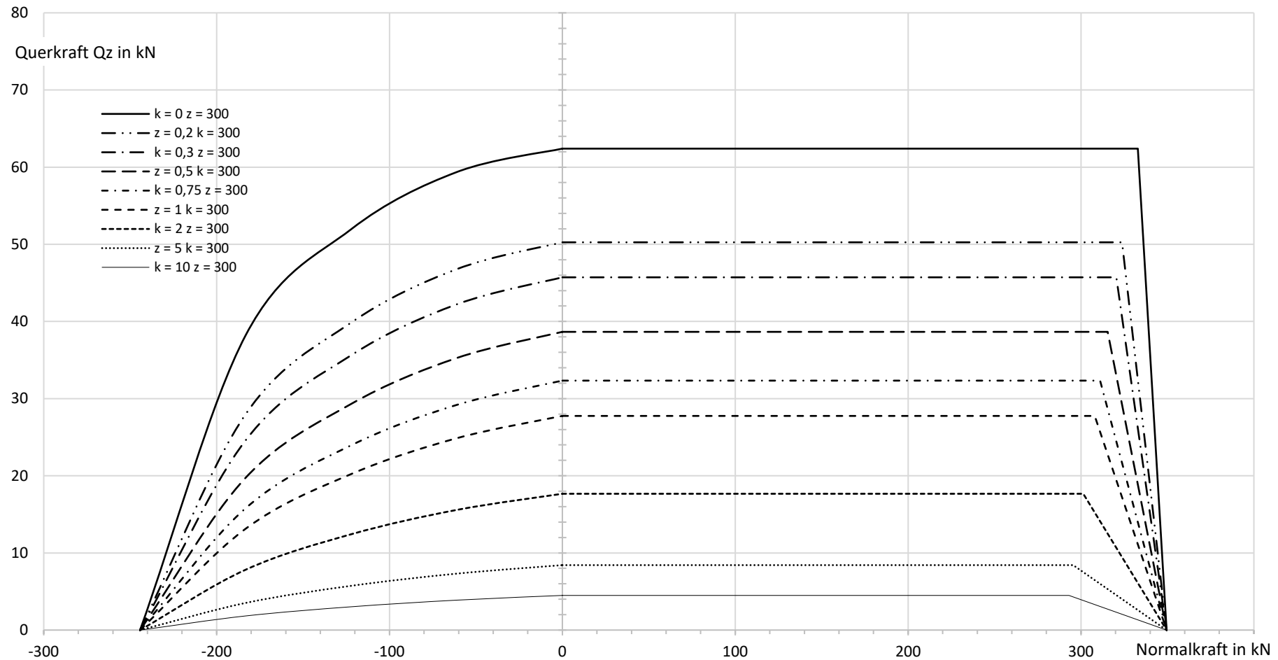
Abb. 12: Querkraft in z-Richtung, FVST 22, z = 300 mm
