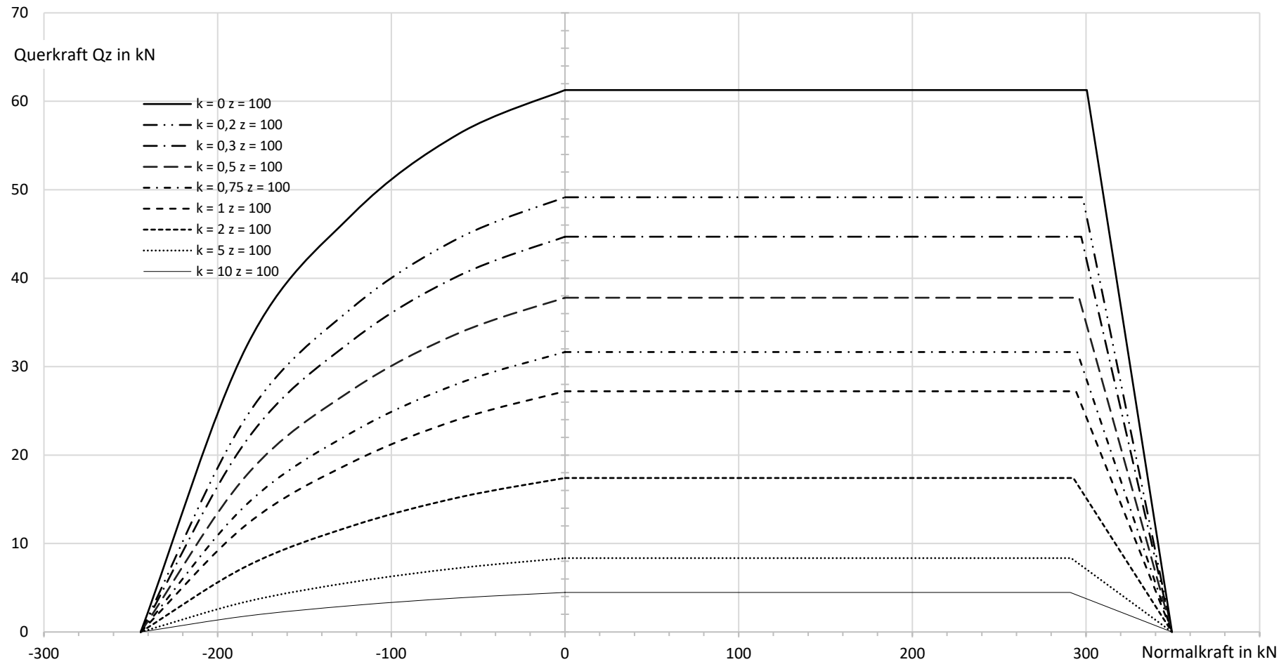
Abb. 11: Querkraft in z-Richtung, FVST 22, z = 100 mm
