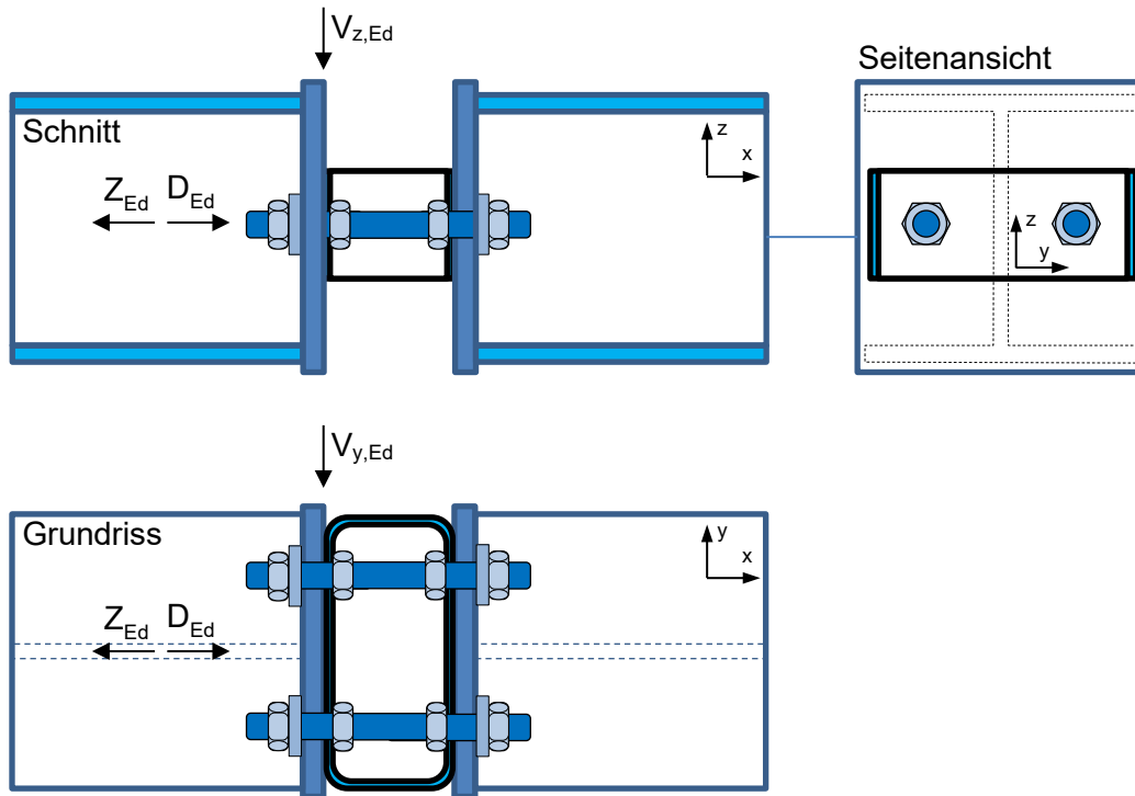
Abb. 2: Ein Modul FVST
