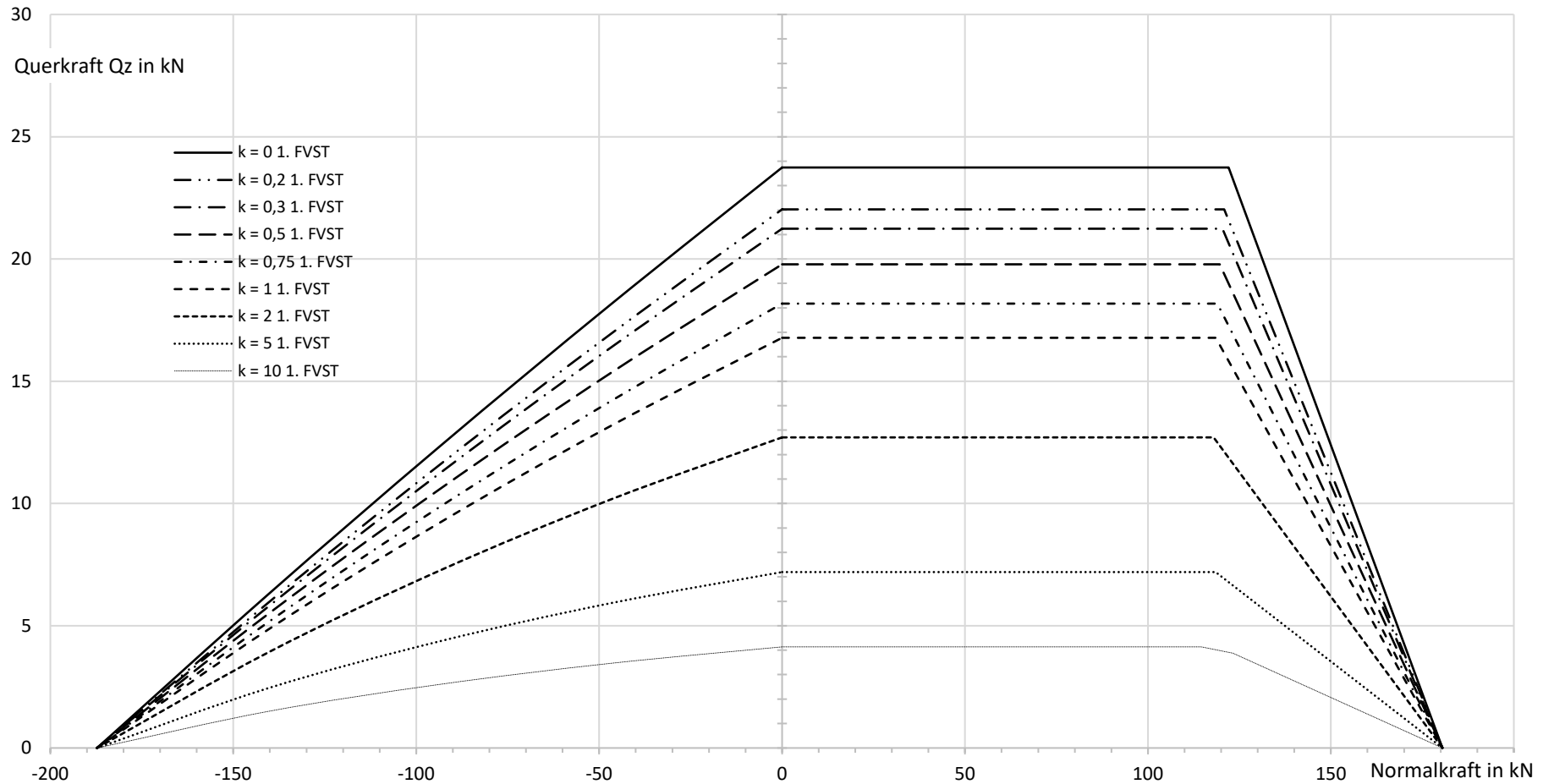
Abb. 5: Querkraft in z-Richtung, ein FVST 16 Modul
