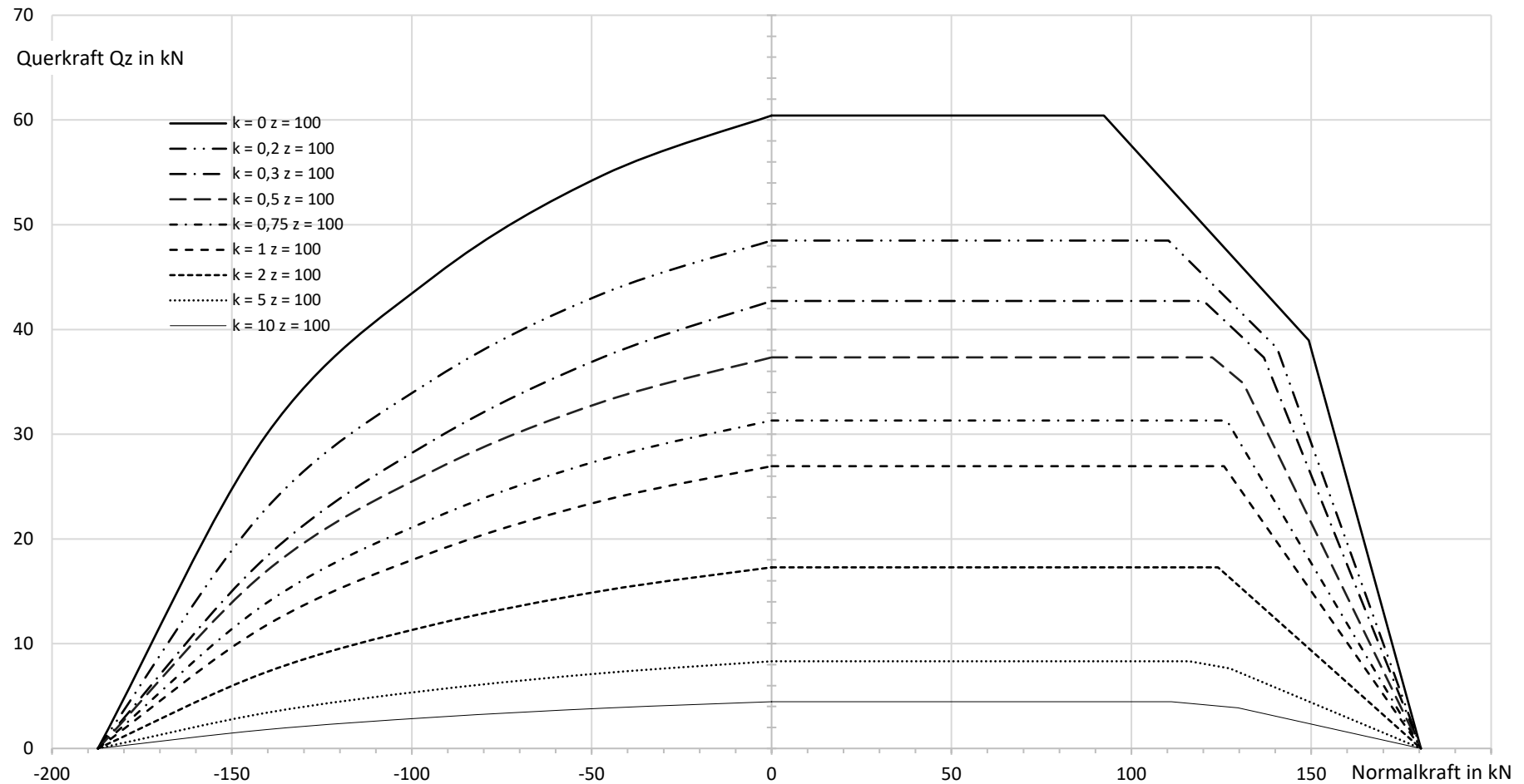
Abb. 7: Querkraft in z-Richtung, FVST 16, z = 100 mm
