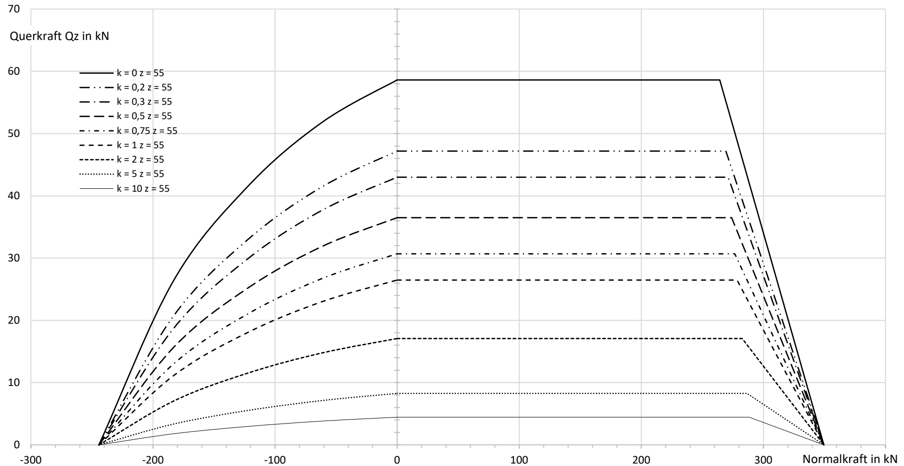
Abb. 10: Querkraft in z-Richtung, FVST 22, z = 55 mm
