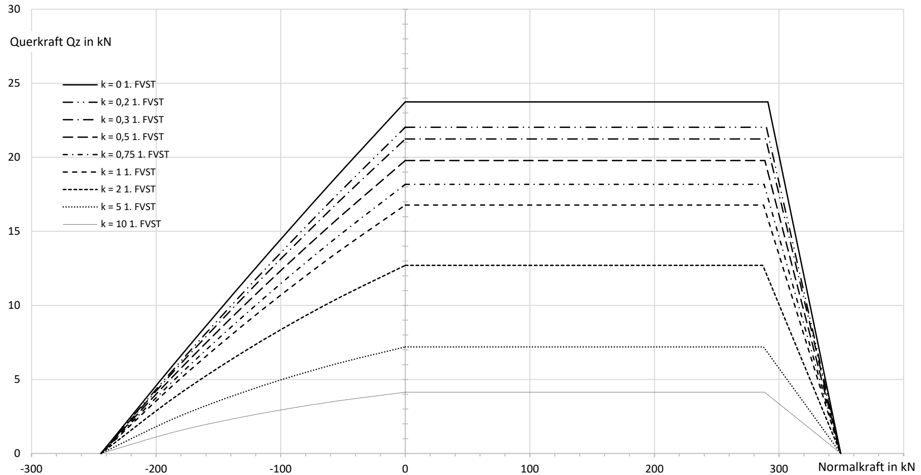
Abb. 9: Querkraft in z-Richtung, FVST 22, ein Modul
